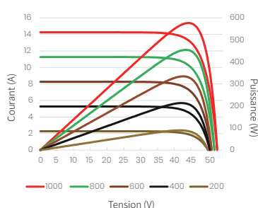
Courbes courant-tension et puissance-tension (585W)
